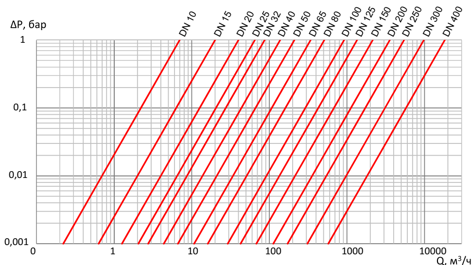
ДИАГРАММА ПОТЕРИ ДАВЛЕНИЯ ДЛЯ ПРОХОДНЫХ КРАНОВ
